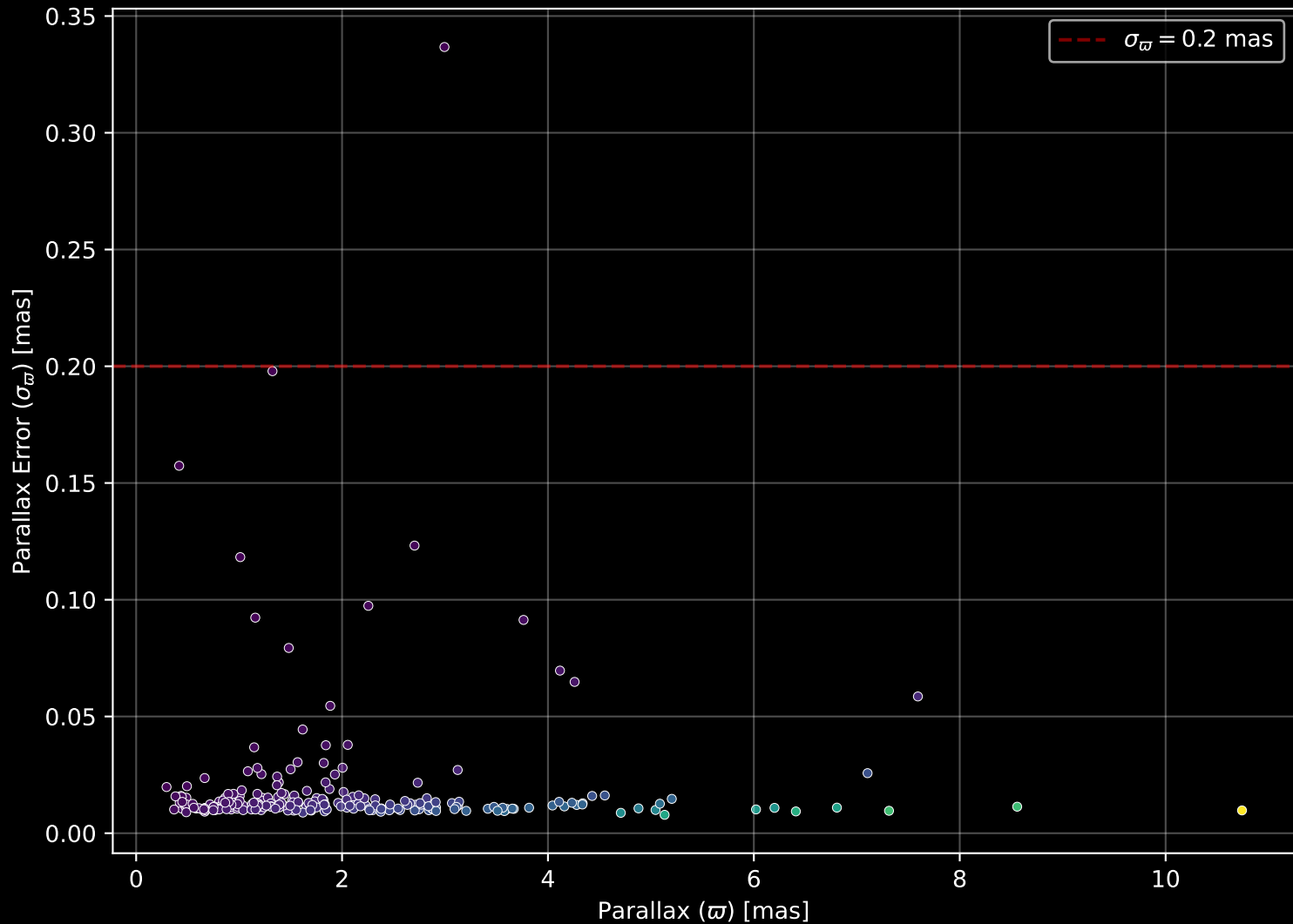
GALAH DR4 Field: [7194] Parallax Quality (n= 233)
