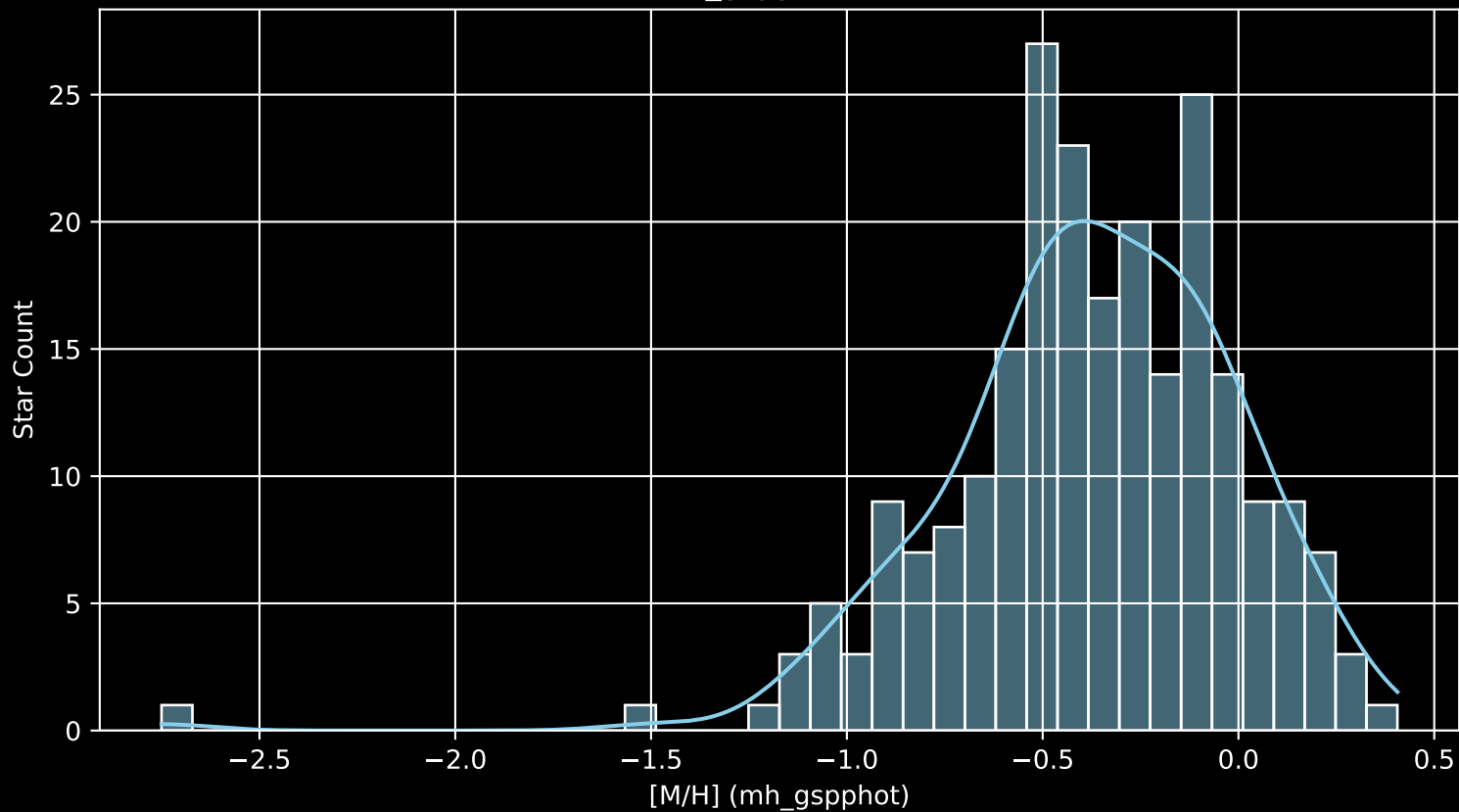
GALAH DR4 Field: [7194] [M/H] (mh_gspphot) (n= 232)
