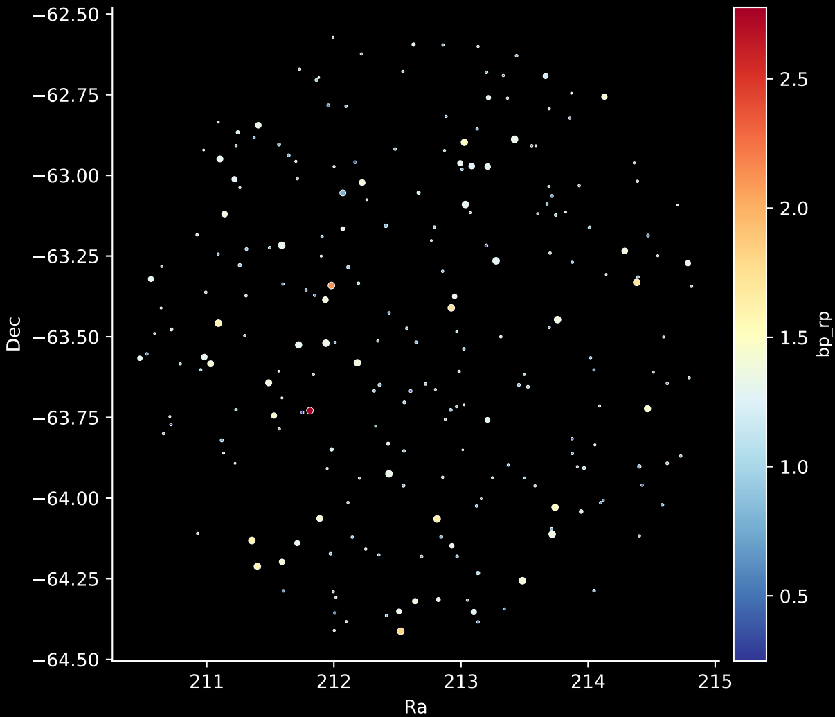
GALAH DR4 Field: [7194] Stars: 233
